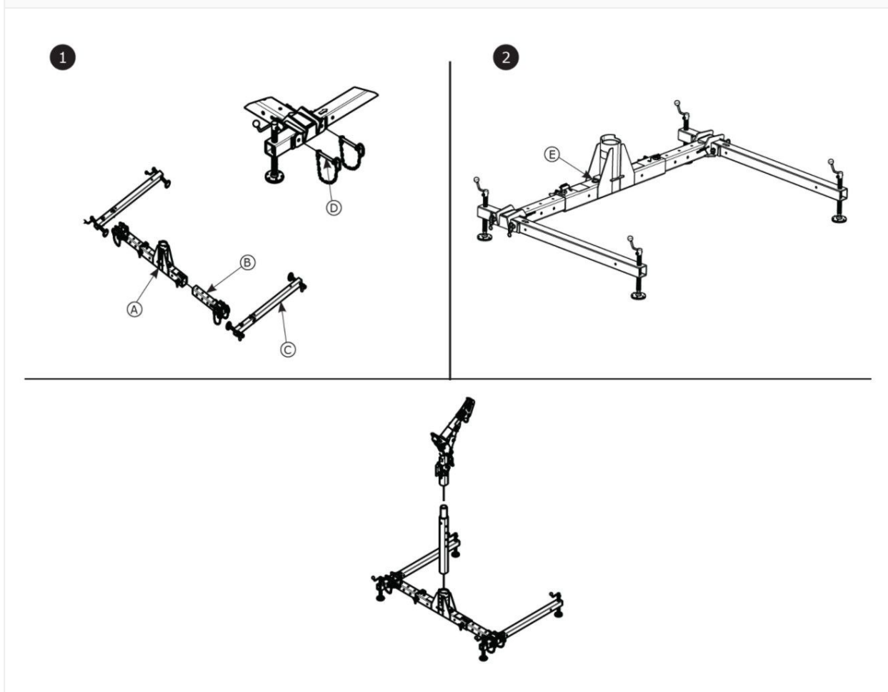
Imagem 6 - Instalar a base de braço elevatório
