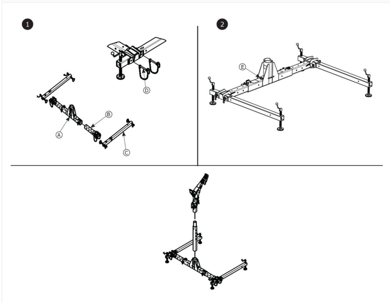
Figure 6 : installation de la base de bossoir
