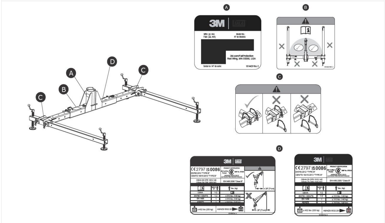
그림 7- 제품 라벨
