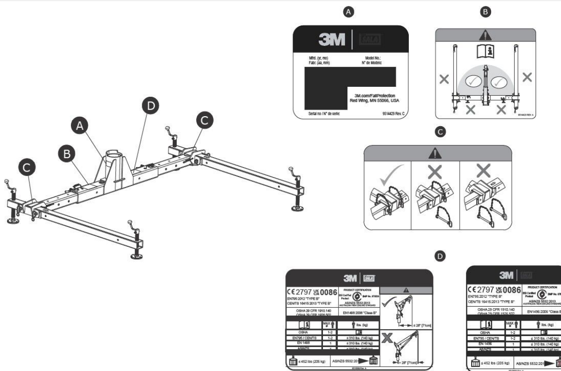
Slika 7 – Oznake izdelka
