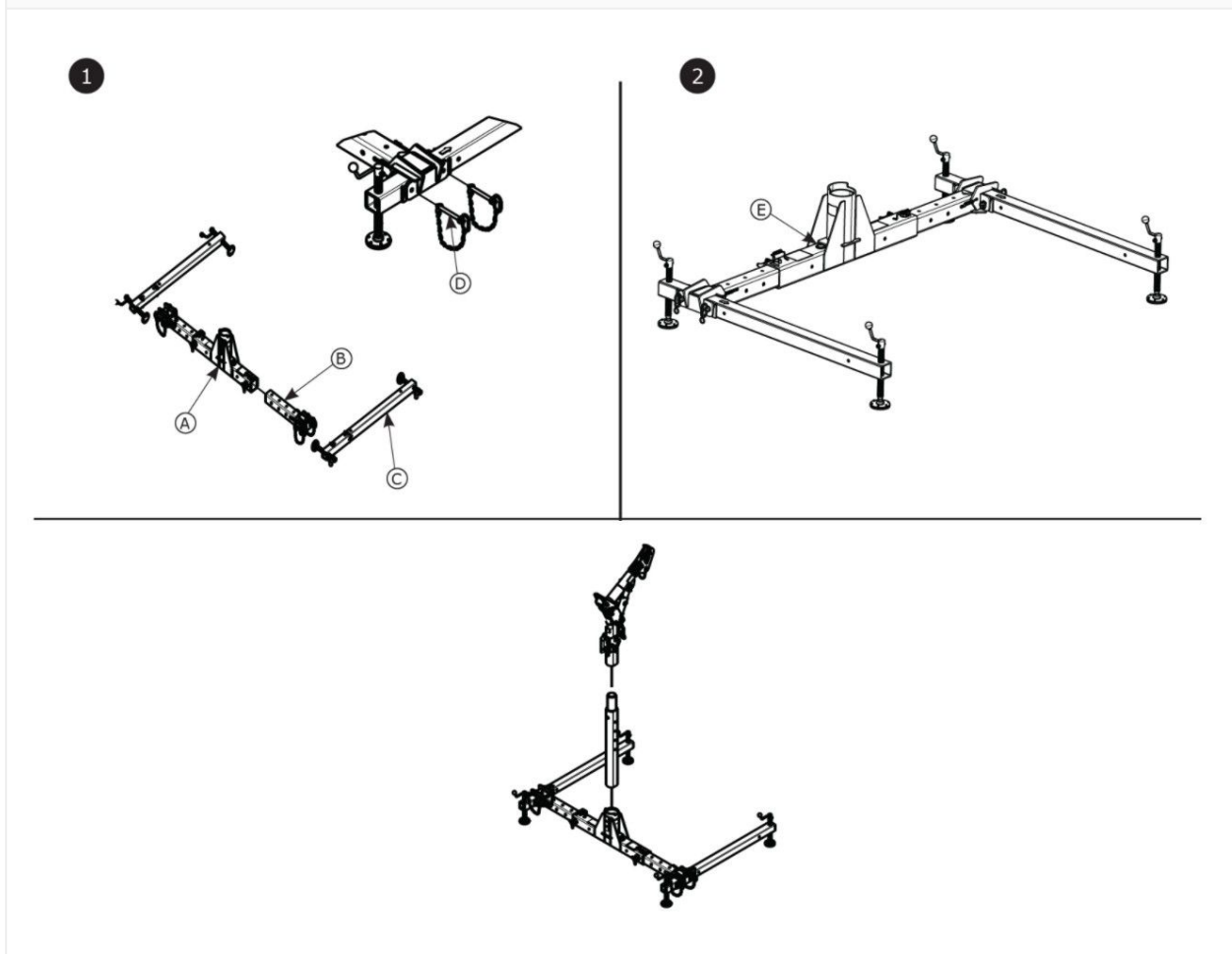
Abbildung 6 – Montage des Auslegersockels
