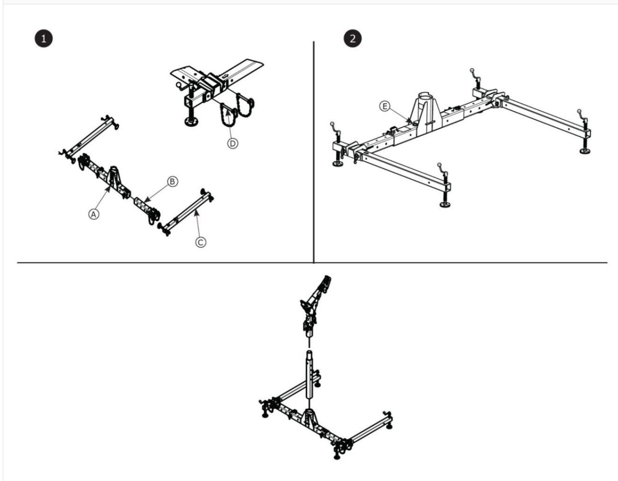
Figure 6 : installation de la base de potence
