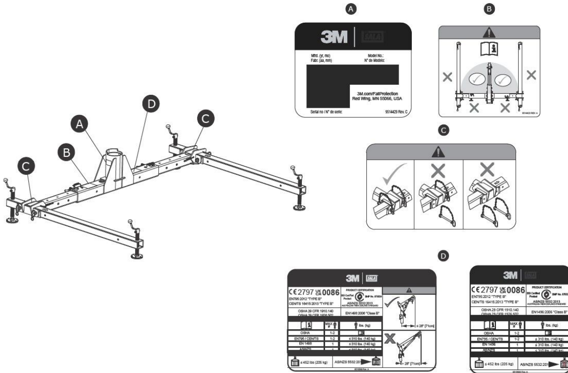
Kuva 7 – Tuotetarrat
