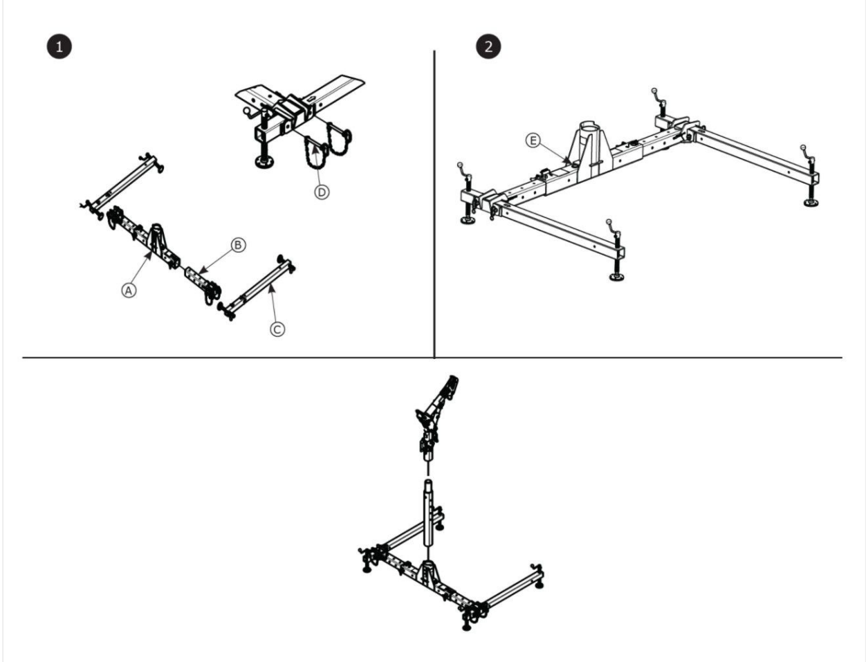
Figura 6: Instalación de la base del pescante
